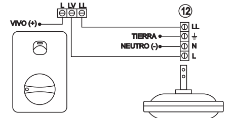
Fig 4 "Conexión eléctrica"
