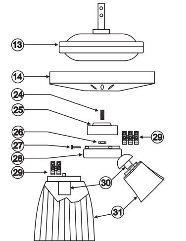
Fig 5 "Conexión de la luminaria"
